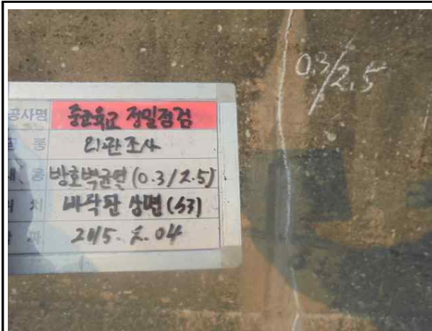
방호벽 S3 c/w=0.3mm이상 균열
