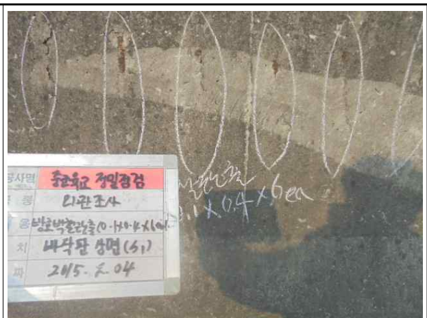
방호벽 S1 철근노출
