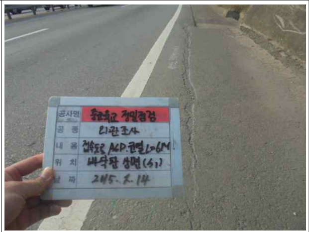
광양방향 S1 접속도로 교면포장 균열
