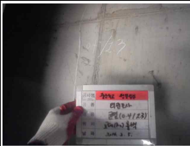
A2 교대 홍벽 c/w=0.4mm 균열
