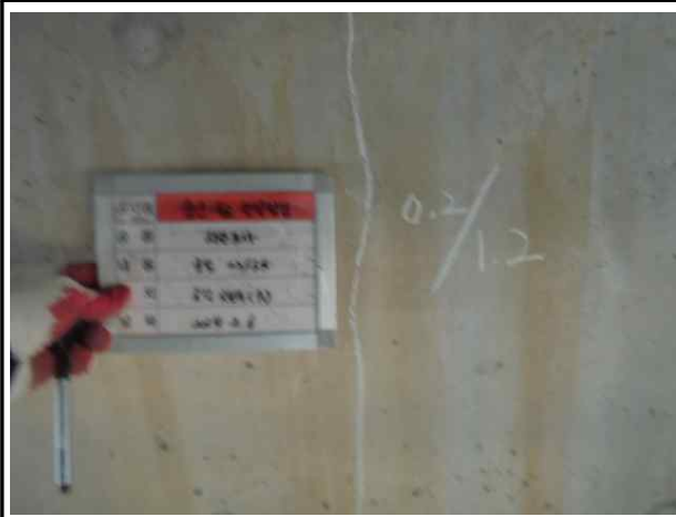
P1 코핑부 c/w=0.2mm 균열
