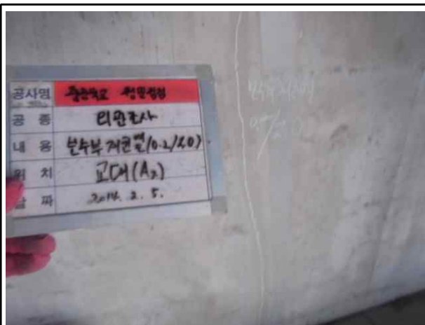
A2 교대 보수부 재균열(c/w=0.2mm)
